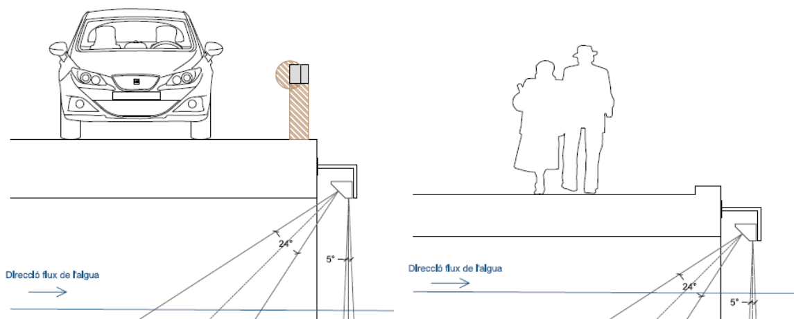
Imatge 20. Ubicació dels sensors en estructures de pas sota camins i carreteres
